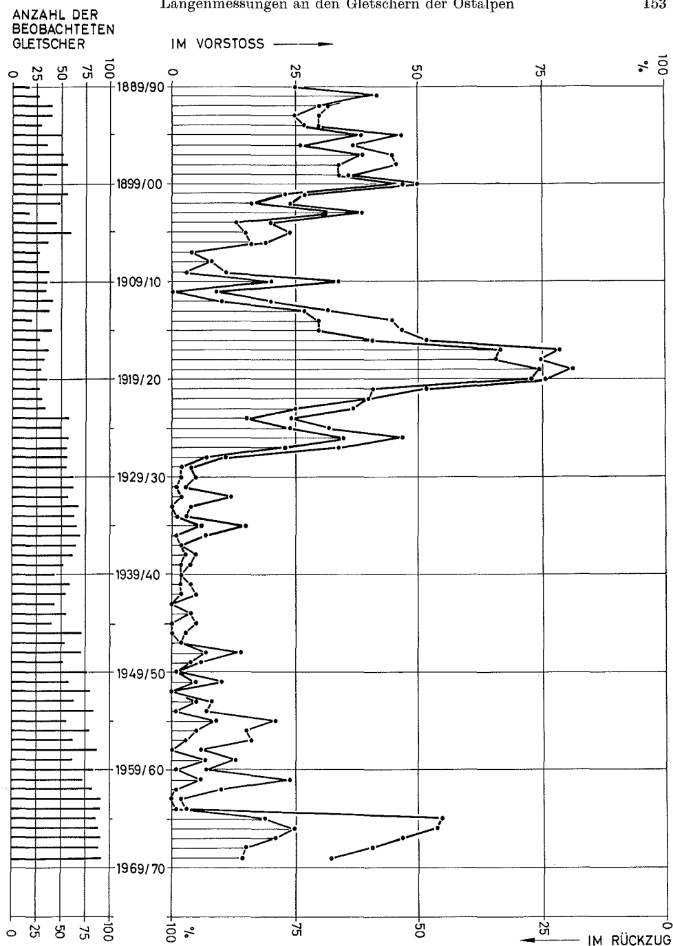
Abb. 1: Die Schwankungen der Gletscherenden in den österreichischen Ostalpen von 1890 bis 1969. Von der Summe der beobachteten Gletscher sind auf der Ordinate die Prozentsätze für Vorstoß (von unten nach oben), für Rückzug (von oben nach unten) und für stationäres Verhalten aufgetragen.
