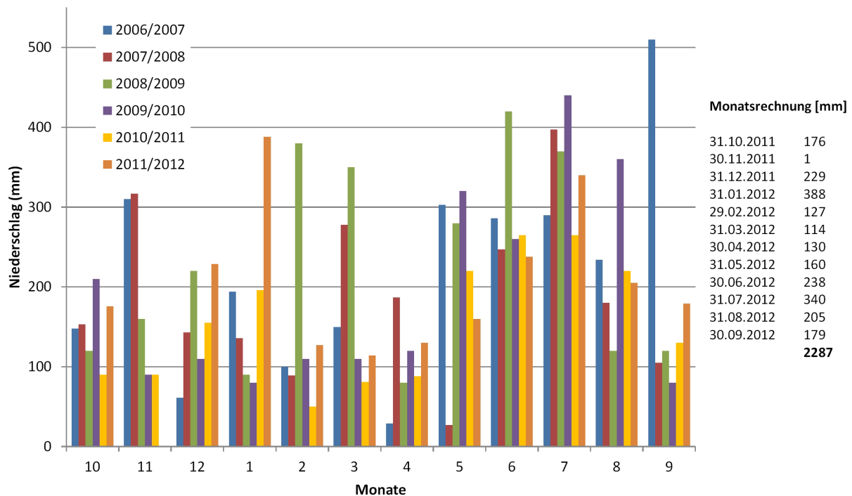
Abbildung 4.2: Vergleich der monatlichen Niederschlagssummen der Haushaltsjahre 2006/07 bis 2011/12 sowie die Messwerte des Totalisators 2011/12 in mm.
