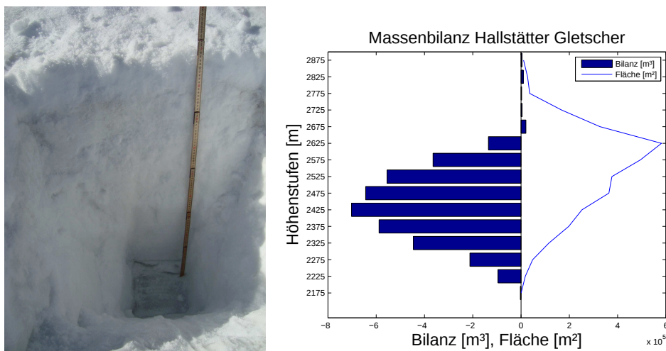
Abbildung 0.1: Der Schneeschacht 3a am 04.10.2012 (links); Massenbilanz und Verteilung der Fläche des Hallstätter Gletschers nach Höhenstufen 2011/12 (rechts).
