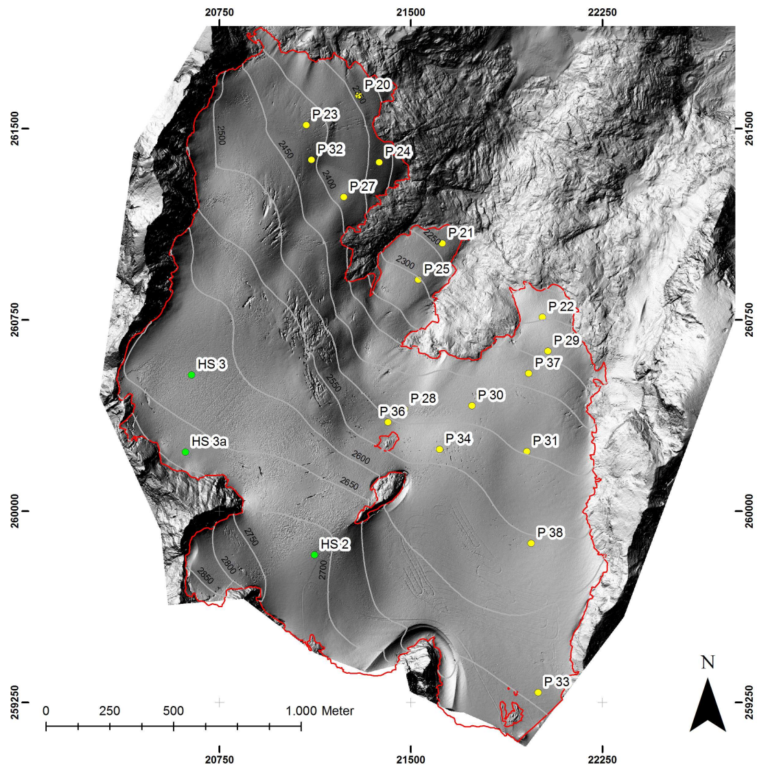
Abbildung 4.1: Positionen der Pegel und Schächte 2011/12 mit 50 m Höhengichtlinien und Gletschergrenze 2009 (rot). Kartengrundlage beleuchtetes Höhenmodell aus Laserscandaten (2007) in Gauß Krüger Koordinaten A31.
