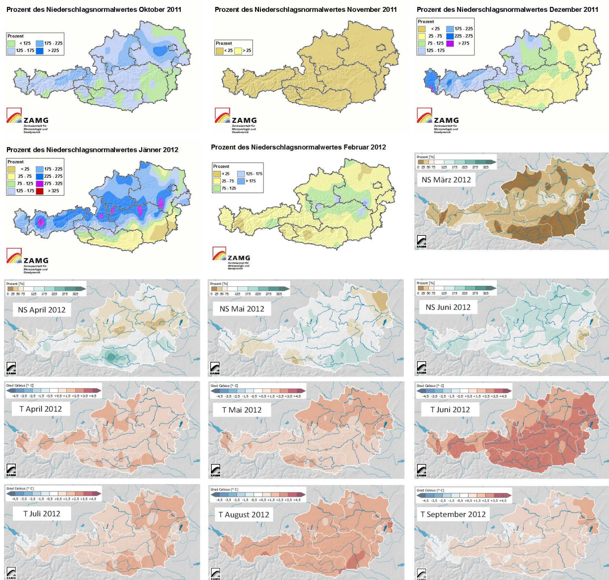
Abbildung 3.2: Übersicht der Abweichungen vom langjährigen Mittel des Niederschlags und der Temperatur (Mittel bezogen auf die Periode 1971 bis 2000). Die Abbildungen werden von der ZAMG unter www.zamg.ac.at zur Verfügung gestellt.
