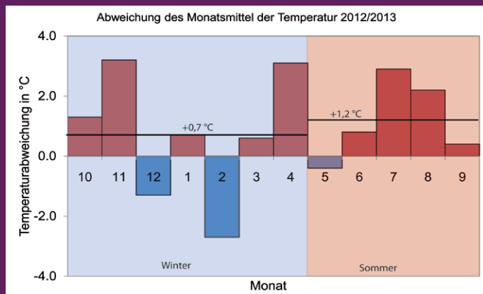
Abbildung 2: Abweichungen der monatlichen und jahreszeitlichen Lufttemperaturen 2012/2013 vom Mittel 1960–1990 an den Bergstationen Sonnblick, Säntis und Zugspitze.
