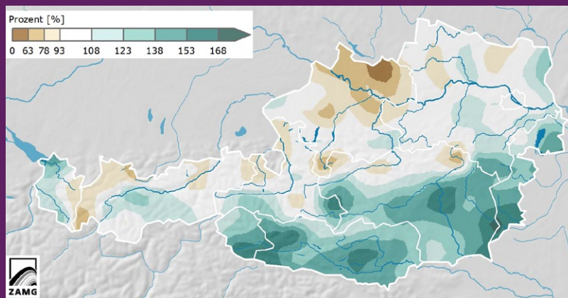
Abbildung 1: Die Abweichung des Niederschlags der Wintermonate 2012/2013 vom langjährigen Mittel 1971–2000 (Quelle: www.zamg.ac.at )
