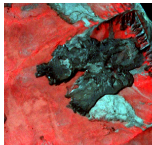
Planet
