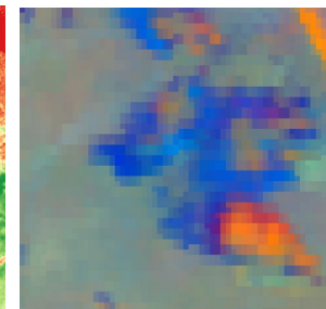
Landsat Trends
